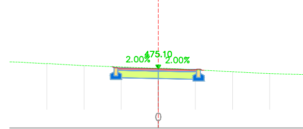
PP 3 – 0+030.00
