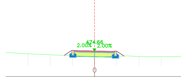
PP 1 – 0+003.00
